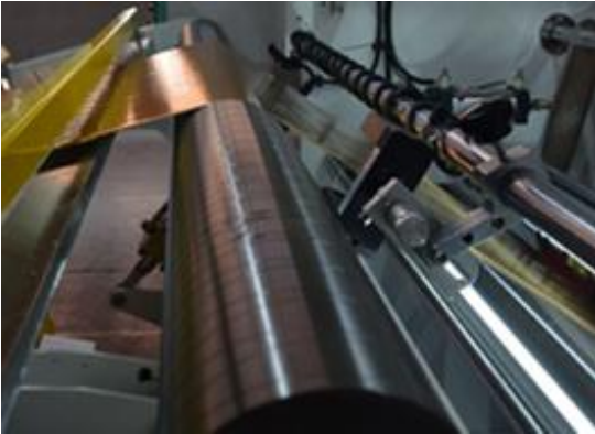
Ultrasonic Edge Guider ST
